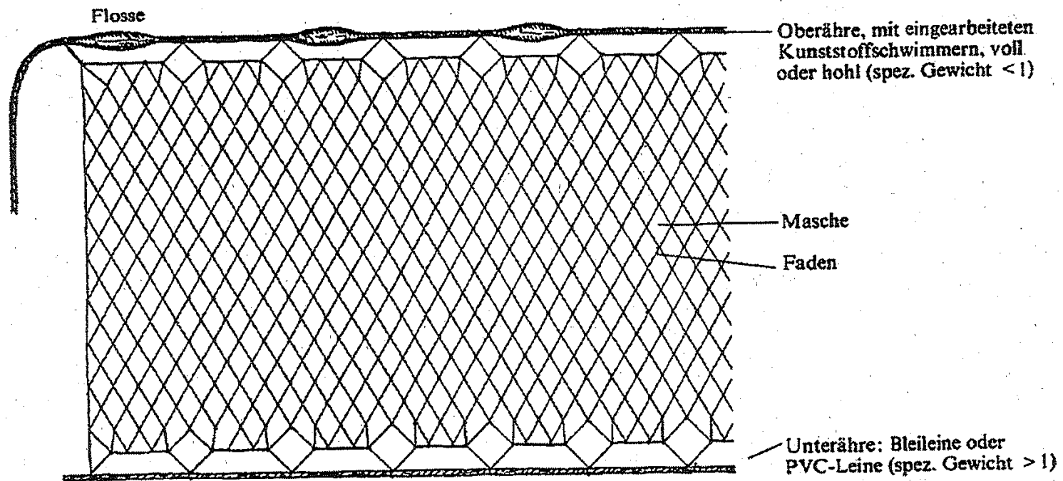
Fig. 2: Benennung der einzelnen Teile eines Kiemennetzes (Maschenreihe, Maschenschenkel, Schnur)
