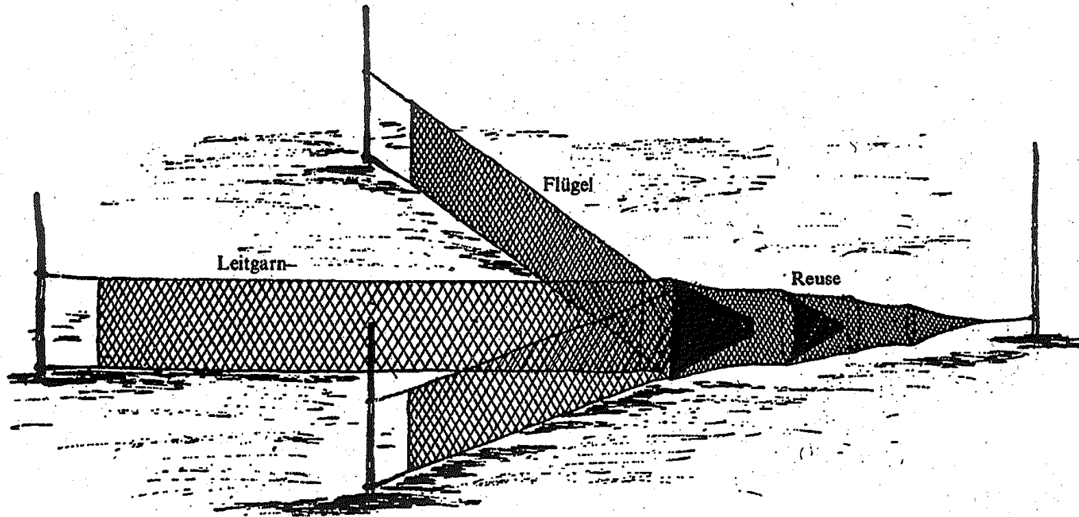
Fig. 7: Einzelne Aalreuse mit Flügeln und Leitgarn
